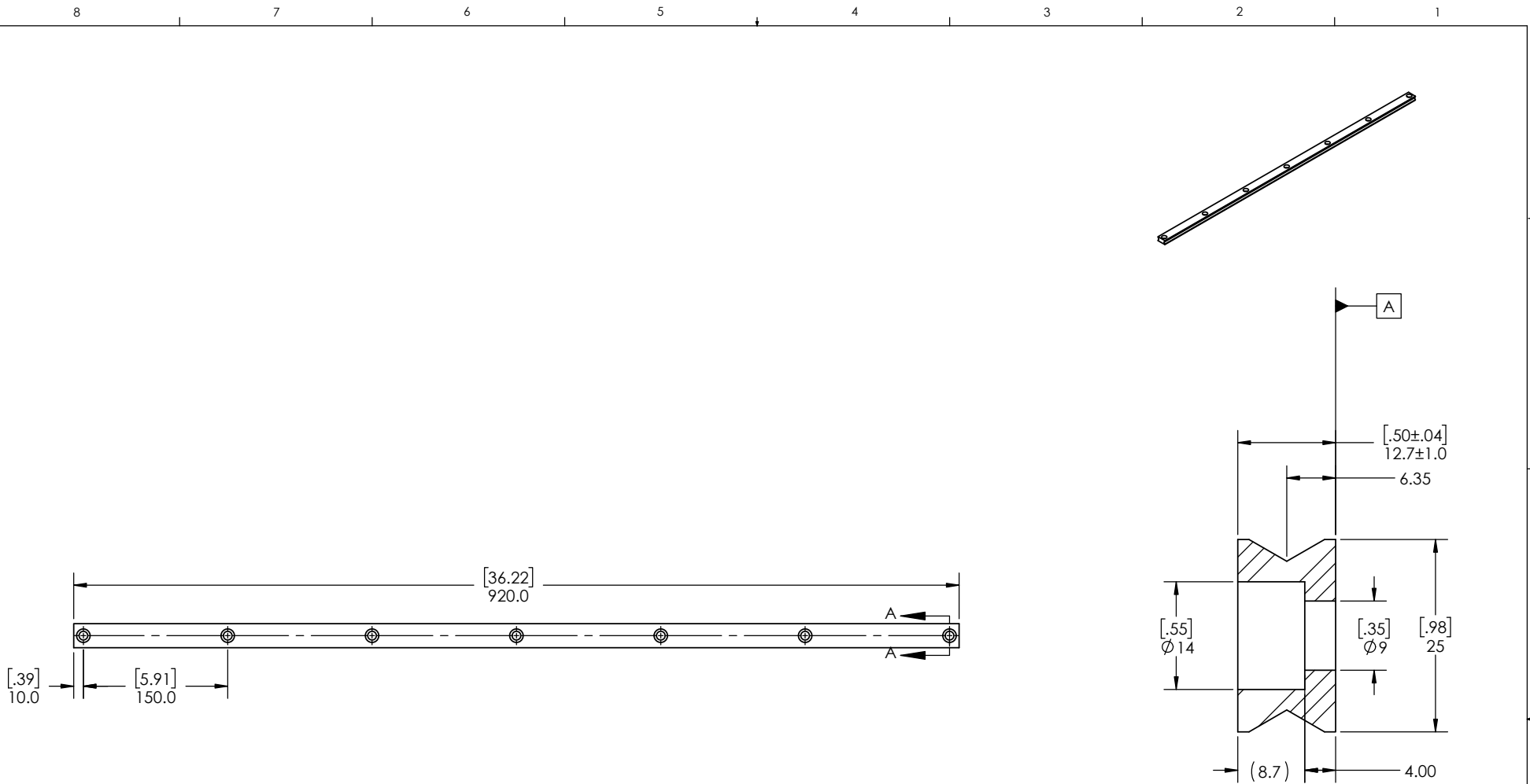
SECTION A-A SCALE 2 : 1
